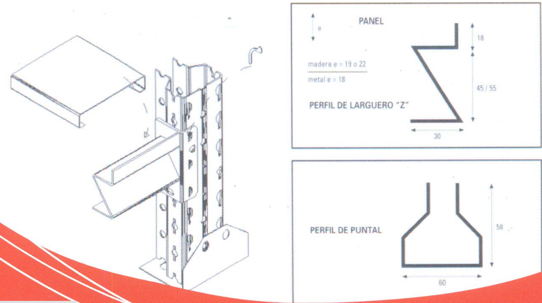
Travesaño de apoyo
