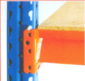
Panel aglomerado
